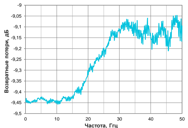
Возвратные потери
