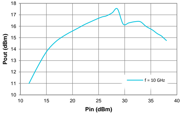
Pout
