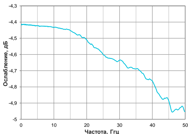
Ослабление
