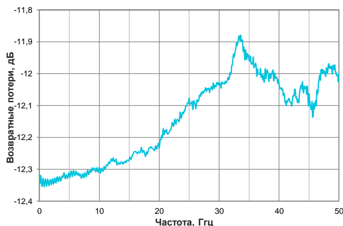
Возвратные потери
